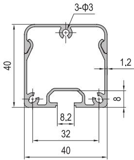
Conduit Profile-40x40
