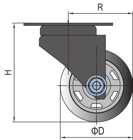
Castor-Plate-Fixed
