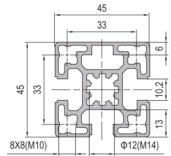
45x45 3 slots
