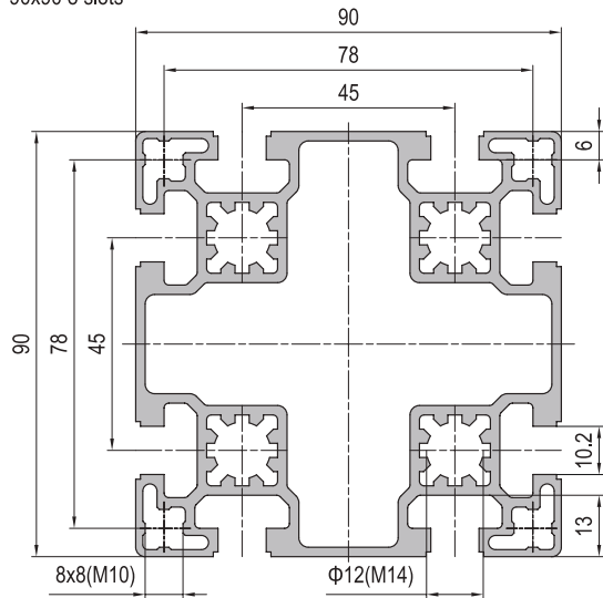
90x90 8 slots
