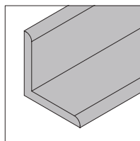
Angle Profile 30x30x4
