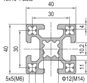
40x40 4 slots
