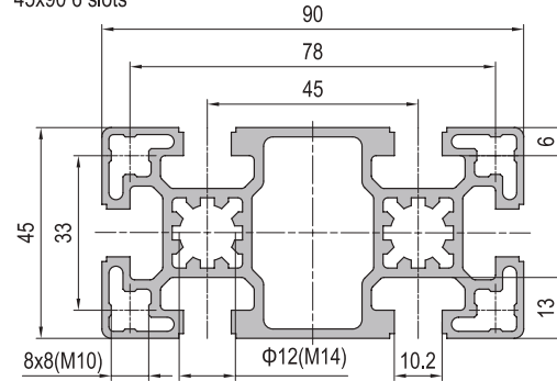
45x90 6 slots
