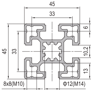
45x45 4 slots
