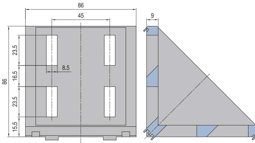
PG45-90x90
