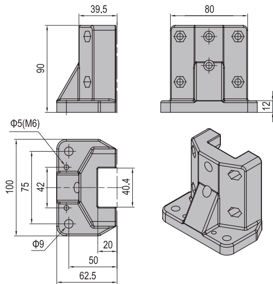
Base Plate-40-B
