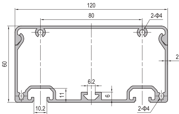
Conduit Profile-60x120
