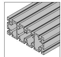
80x200 14 slots
