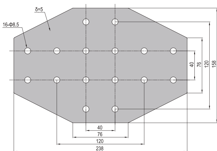
PG40-8080-03
