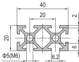
20x40 6 slots
