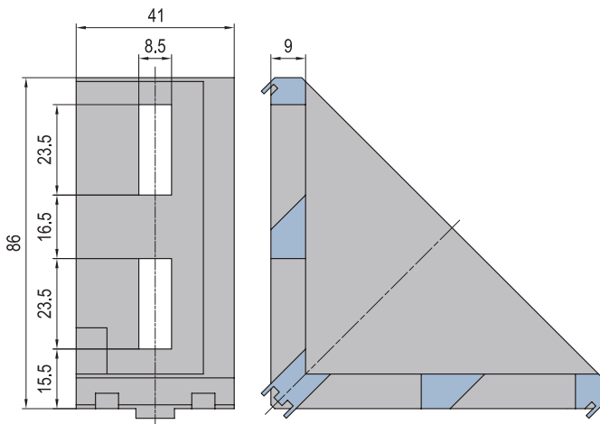
PG45-45x90
