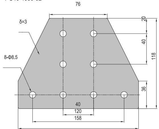
PG40-4080-02
