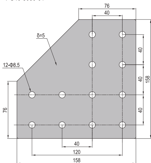
PG40-8080-01
