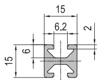
15x15 2 slots
