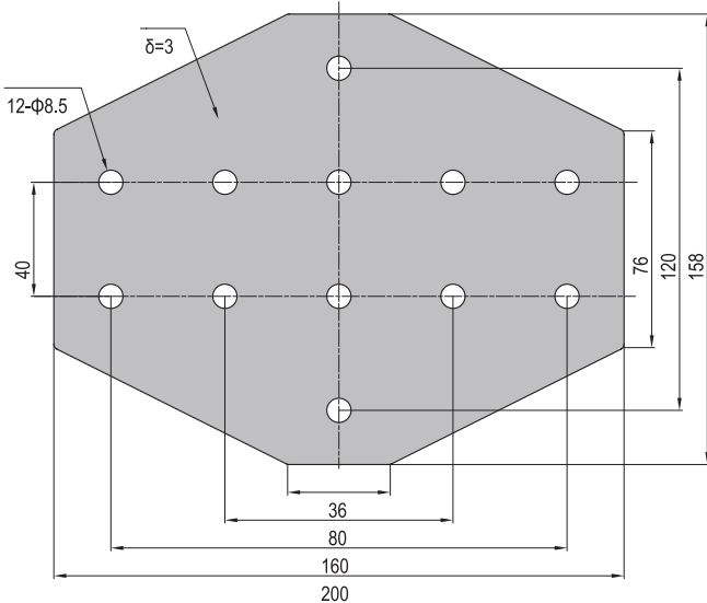
PG40-4080-03
