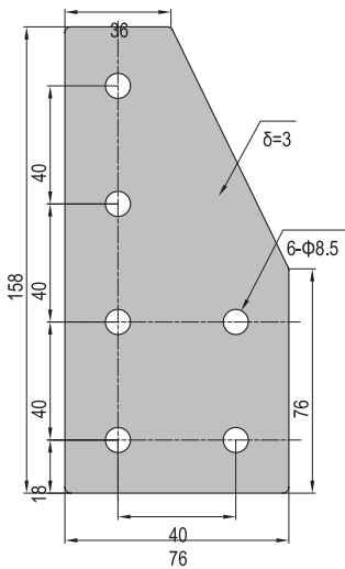
PG40-4080-03
