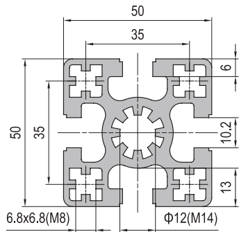
50x50 4 slots
