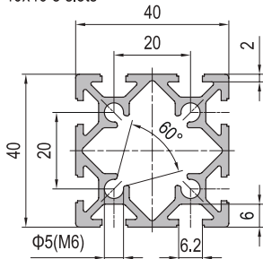
40x40 8 slots
