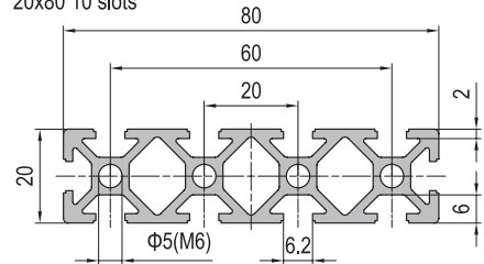
20x80 10 slots
