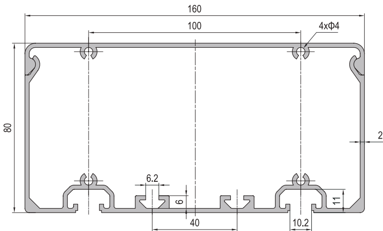
Conduit Profile-80x160
