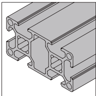
30x60 6 slots
