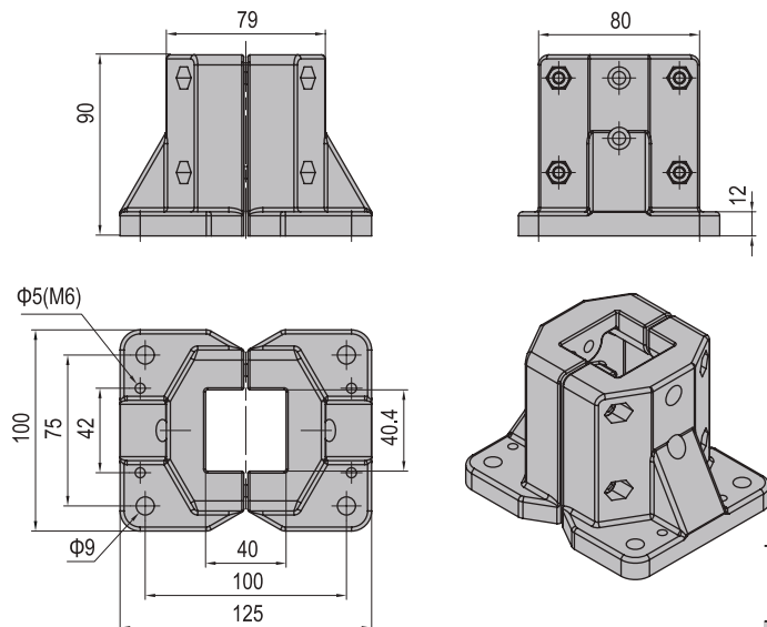
Base Plate-40-B
