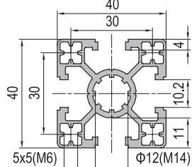
40x40 2 slots Type B
