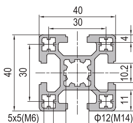
40x40 4 slots
