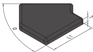
Type E
