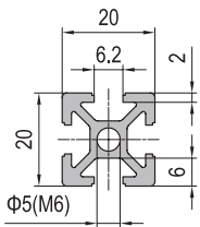
20x20 4 slots
