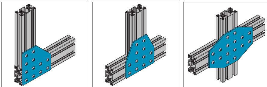
PG40-8080-02
