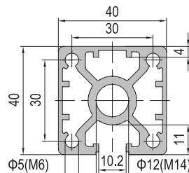
40x40 3 slots
